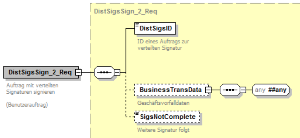
Abbildung 124: Benutzerauftrag Auftrag mit verteilten Signaturen signieren
