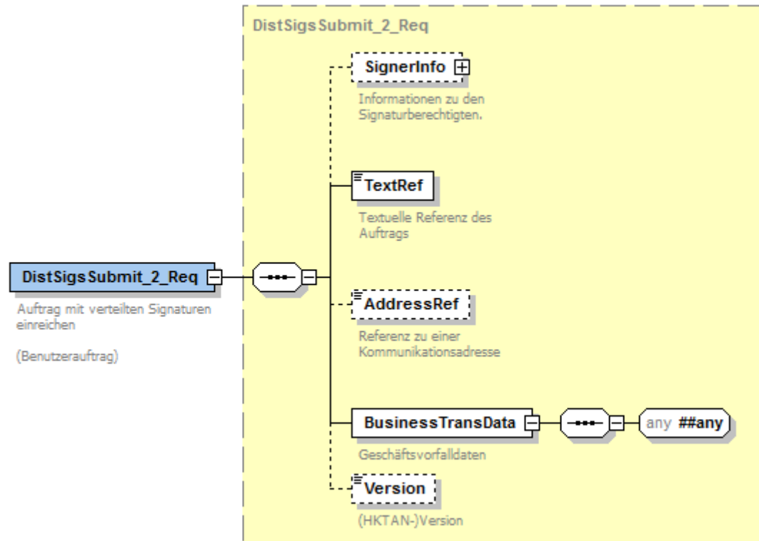
Abbildung 118: Benutzerauftrag Auftrag mit verteilten Signaturen einreichen
