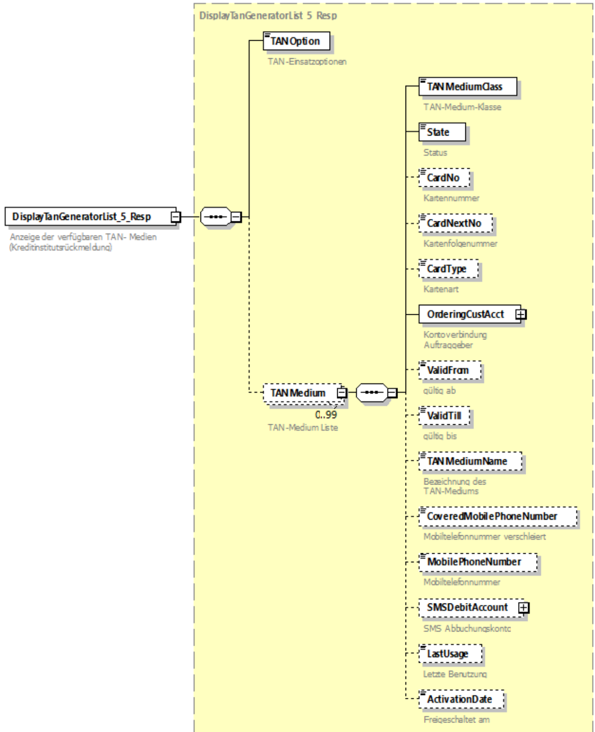
Abbildung 83: Kreditinstitutsrückmeldung Anzeige der verfügbaren TAN-Medien
