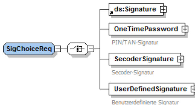
Abbildung 132: Signatur einer Benutzernachricht
