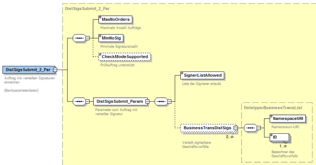
Abbildung 120: Bankparameterdaten Auftrag mit verteilten Signaturen einreichen
