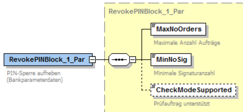
Abbildung 78: Bankparameterdaten PIN-Sperre aufheben
