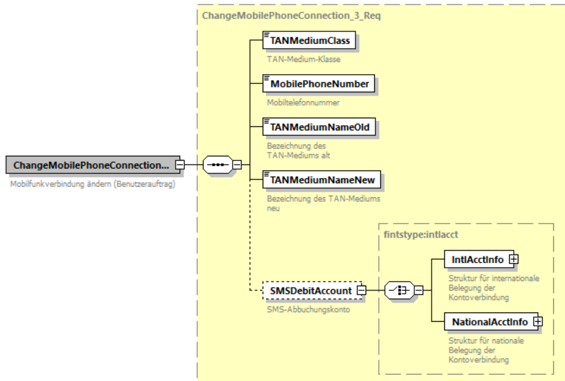
Abbildung 93: Benutzerauftrag Mobilfunkverbindung ändern
