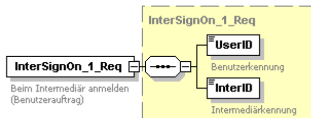
Abbildung 67: Benutzerauftrag Für einen Intermediär anmelden
