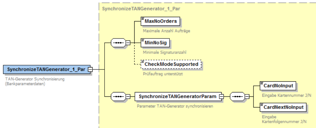
Abbildung 88: Bankparameterdaten TAN-Generator Synchronisierung
