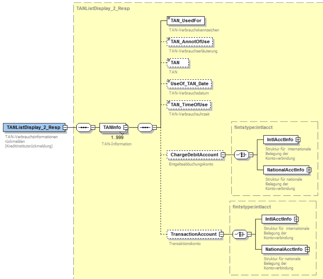
Abbildung 80: Kreditinstitutsrückmeldung TAN-Verbrauchsinformationen anzeigen
