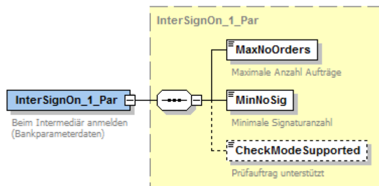
Abbildung 68: Bankparameterdaten Für einen Intermediär anmelden
