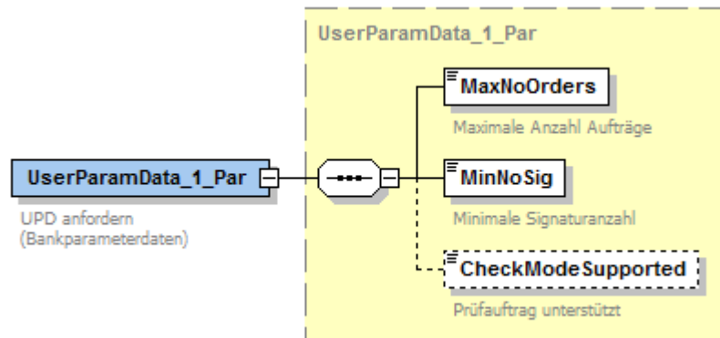
Abbildung 63: Bankparameterdaten UPD anfordern
