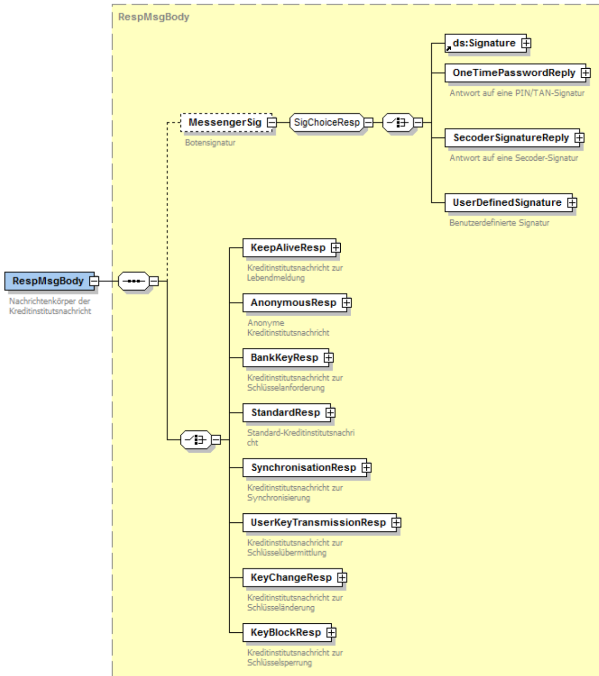
Abbildung 143: Botensignatur im Nachrichtenkörper der Kreditinstitutsnachricht
