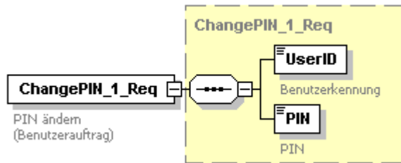
Abbildung 73: Benutzerauftrag PIN ändern
