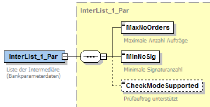
Abbildung 66: Bankparameterdaten Liste der Intermediäre
