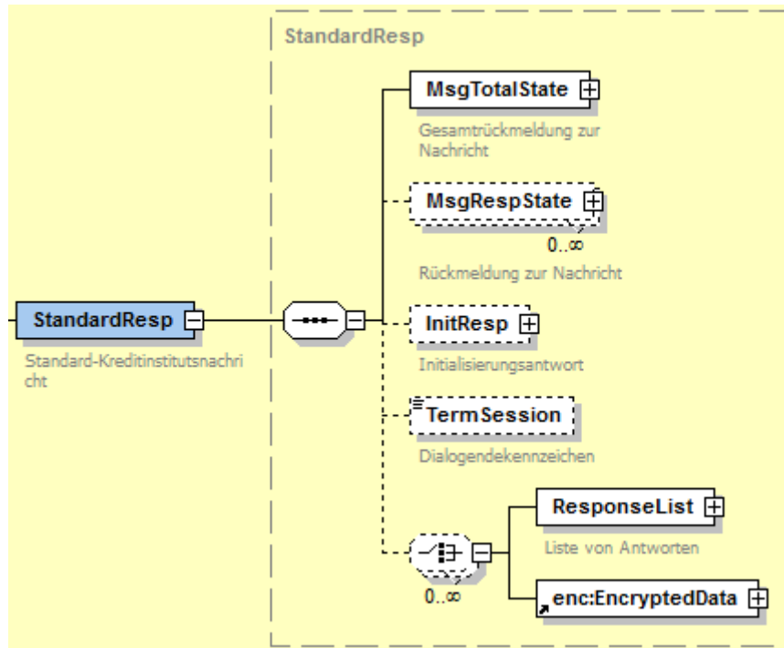
Abbildung 151: Auftragsverschlüsselung in der Standard-Kreditinstitutsnachricht
