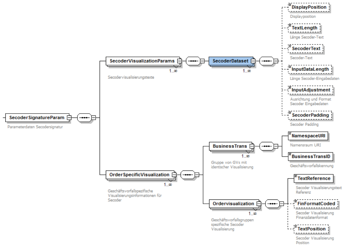
Abbildung 48: Sicherheitsverfahren Secoder – Parameterdaten Secodersignatur
