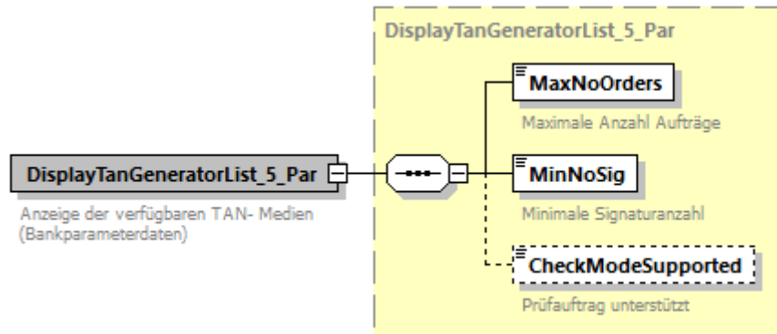
Abbildung 84: Bankparameterdaten Anzeige der verfügbaren TAN-Medien
