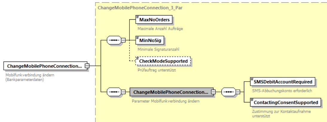
Abbildung 94: Bankparameterdaten Mobilfunkverbindung ändern
