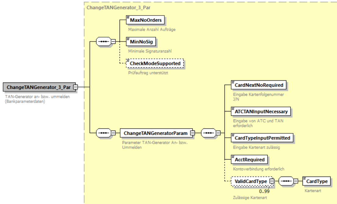
Abbildung 86: Bankparameterdaten TAN-Medium an- bzw. ummelden
