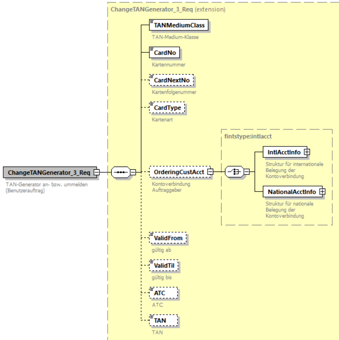
Abbildung 85: Benutzerauftrag TAN-Medium an- bzw. ummelden
