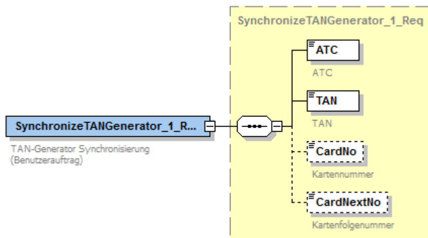
Abbildung 87: Benutzerauftrag TAN-Generator Synchronisierung
