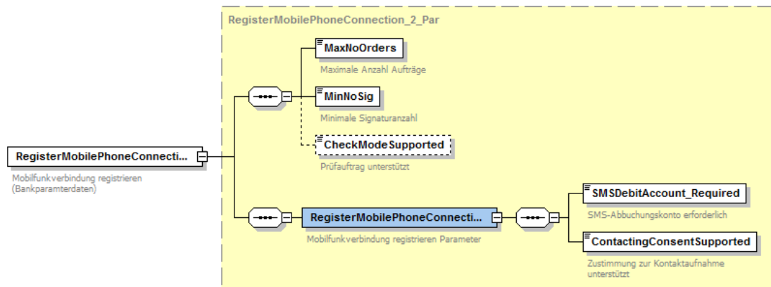
Abbildung 90: Bankparameterdaten Mobilfunkverbindung registrieren
