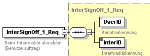
Abbildung 69: Benutzerauftrag Für einen Intermediär abmelden
