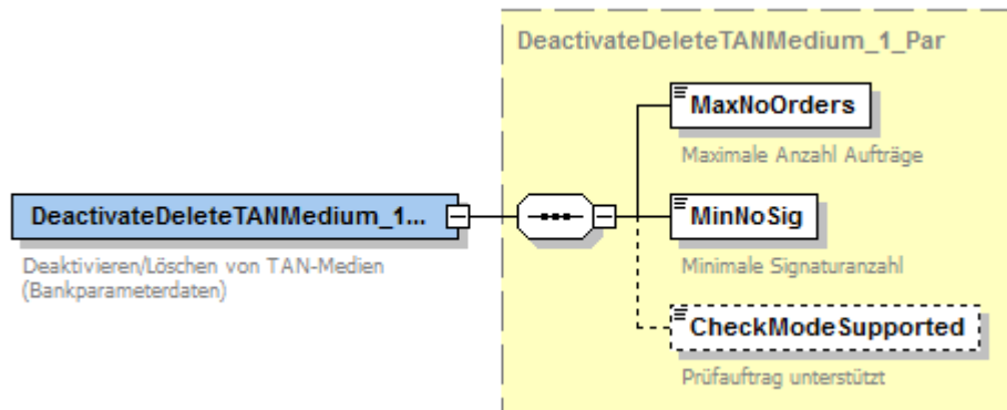
Abbildung 96: Bankparameterdaten Deaktivieren / Löschen von TAN-Medien
