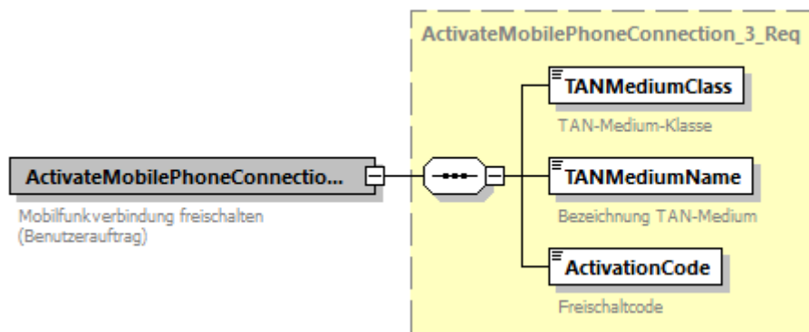
Abbildung 91: Benutzerauftrag Mobilfunkverbindung freischalten
