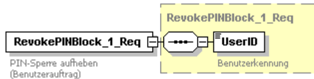
Abbildung 77: Benutzerauftrag PIN-Sperre aufheben
