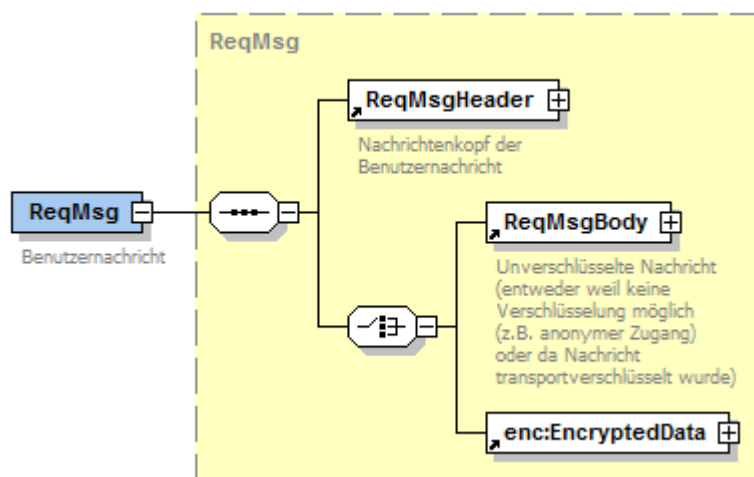
Abbildung 148: Verschlüsselung des Nachrichtenkörpers der Benutzernachricht
