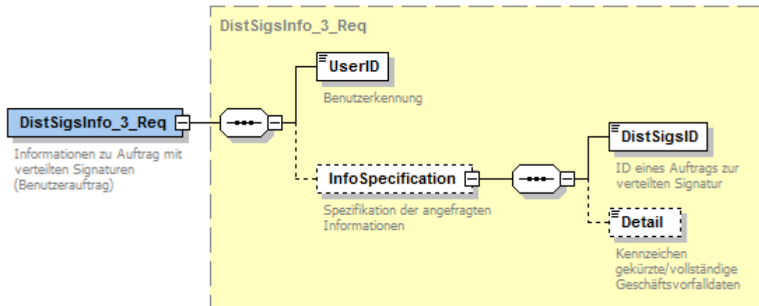
Abbildung 121: Benutzerauftrag Informationen zu Auftrag mit verteilten Signaturen
