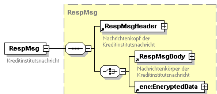
Abbildung 149: Verschlüsselung des Nachrichtenkörpers der Kreditinstitutsnachricht
