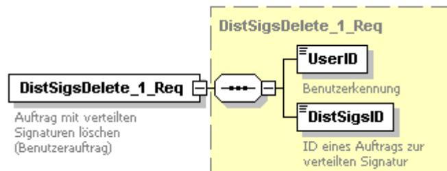
Abbildung 127: Benutzerauftrag Auftrag mit verteilten Signaturen löschen
