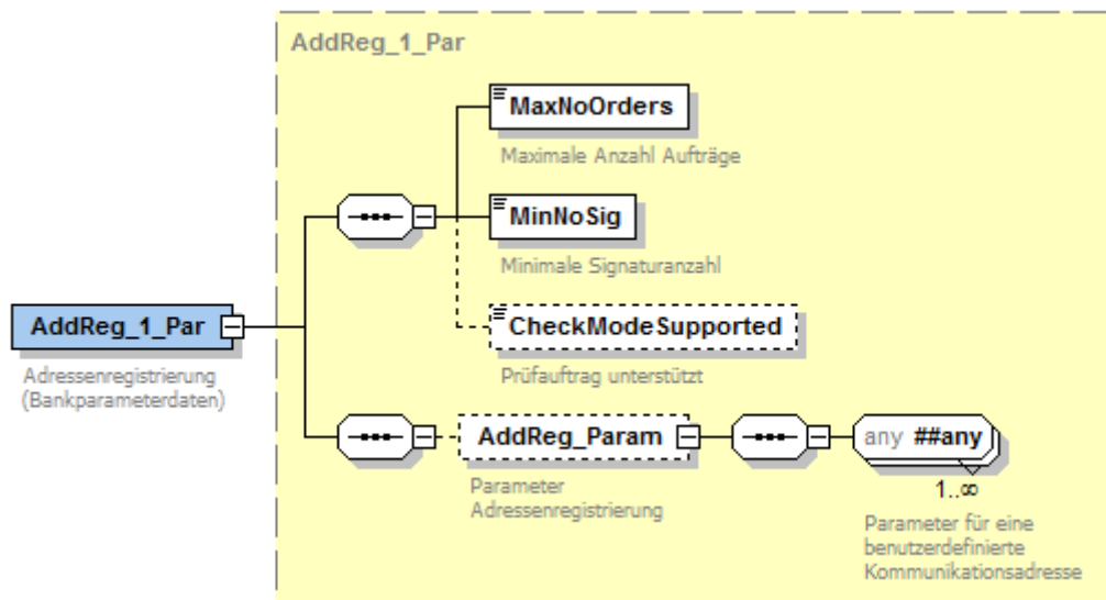
Abbildung 108: Bankparameterdaten Adresse registrieren
