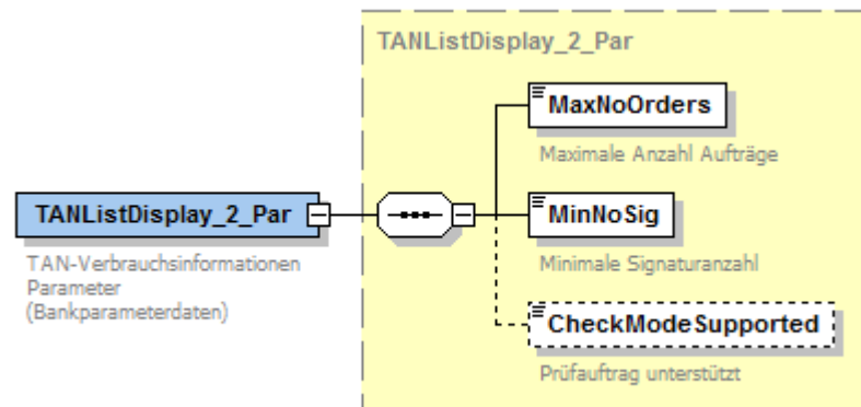
Abbildung 81: Bankparameterdaten TAN-Verbrauchsinformationen anzeigen
