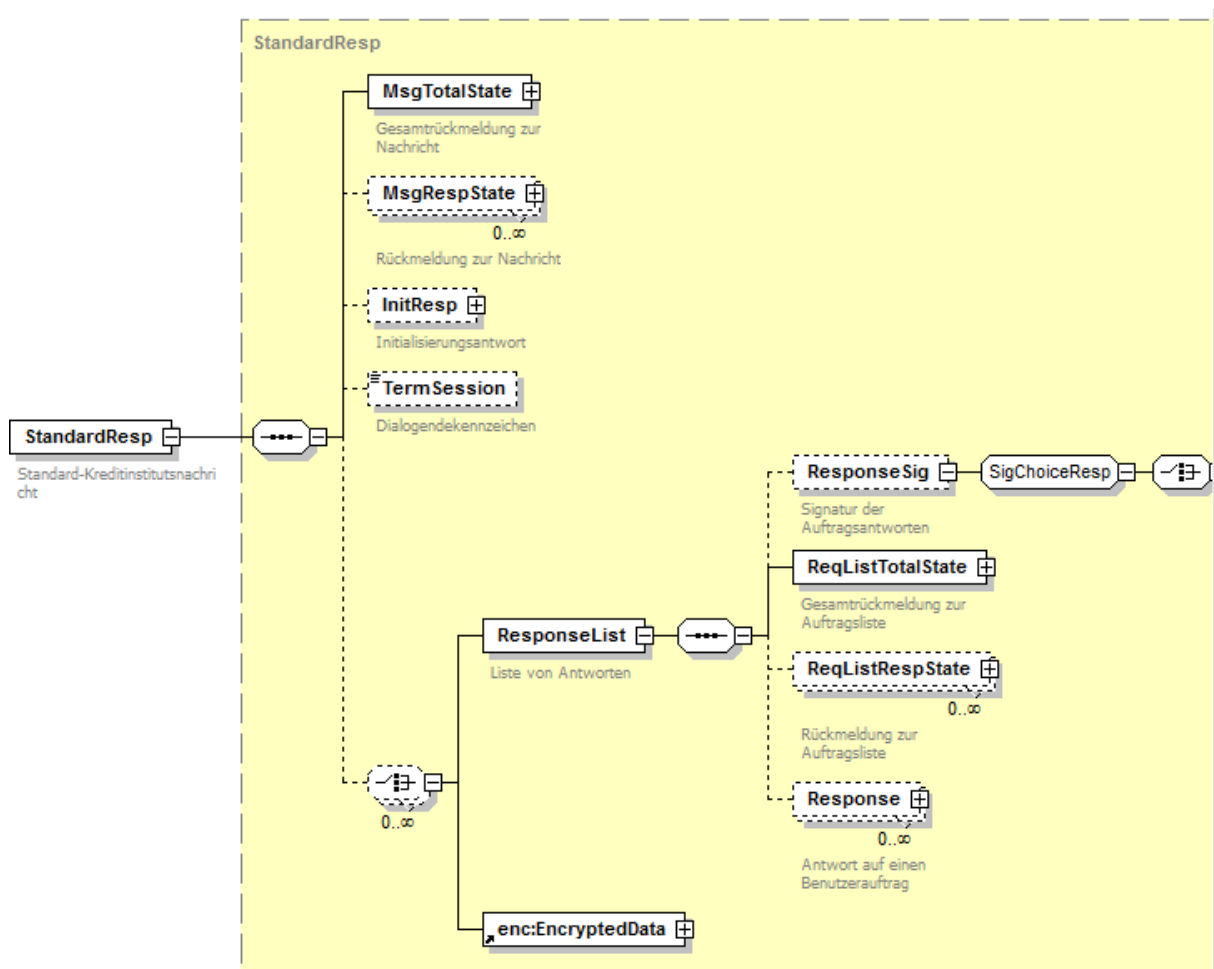
Abbildung 145: Auftragssignatur in einer Kreditinstitutsnachricht
