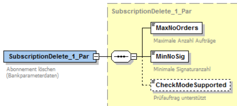
Abbildung 102: Bankparameterdaten Abonnement löschen
