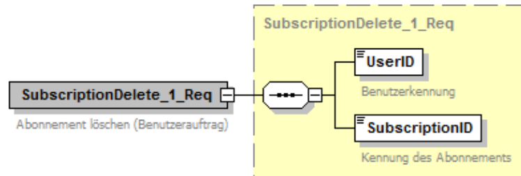
Abbildung 101: Benutzerauftrag Abonnement löschen
