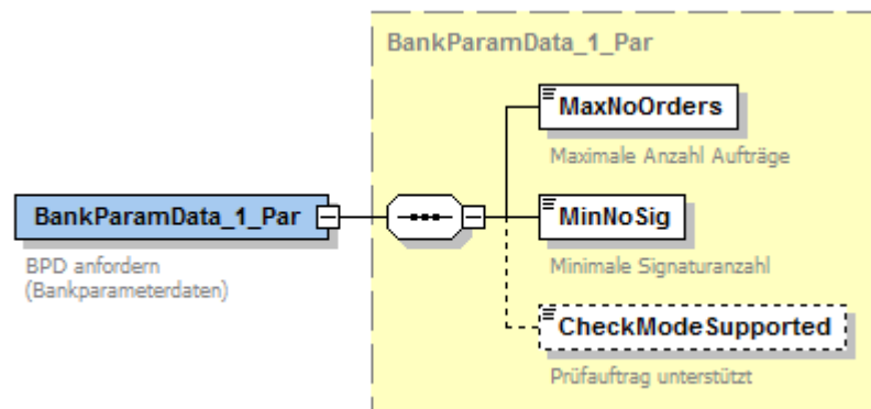
Abbildung 60: Bankparameterdaten BPD anfordern
