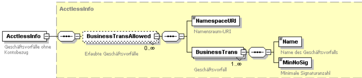
Abbildung 57: Geschäftsvorfälle ohne Kontobezug
