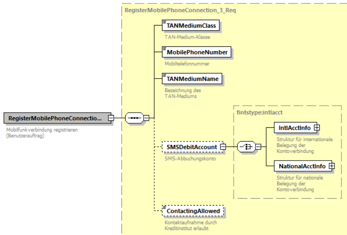
Abbildung 89: Benutzerauftrag Mobilfunkverbindung registrieren
