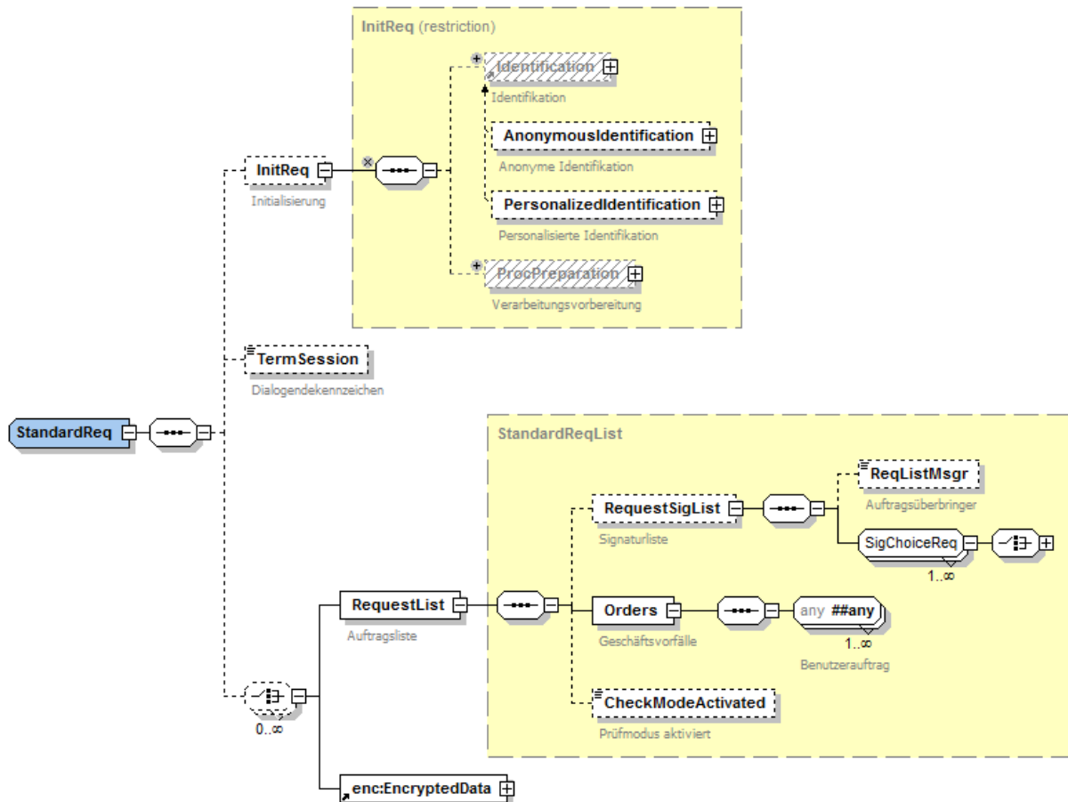
Abbildung 144: Auftragssignatur in einer Benutzernachricht
