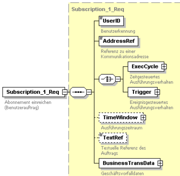
Abbildung 97: Benutzerauftrag Abonnement einreichen
