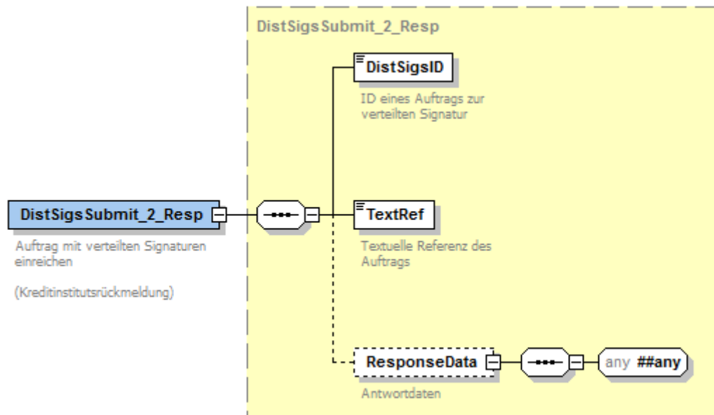
Abbildung 119: Kreditinstitutsrückmeldung Auftrag mit verteilten Signaturen einreichen
