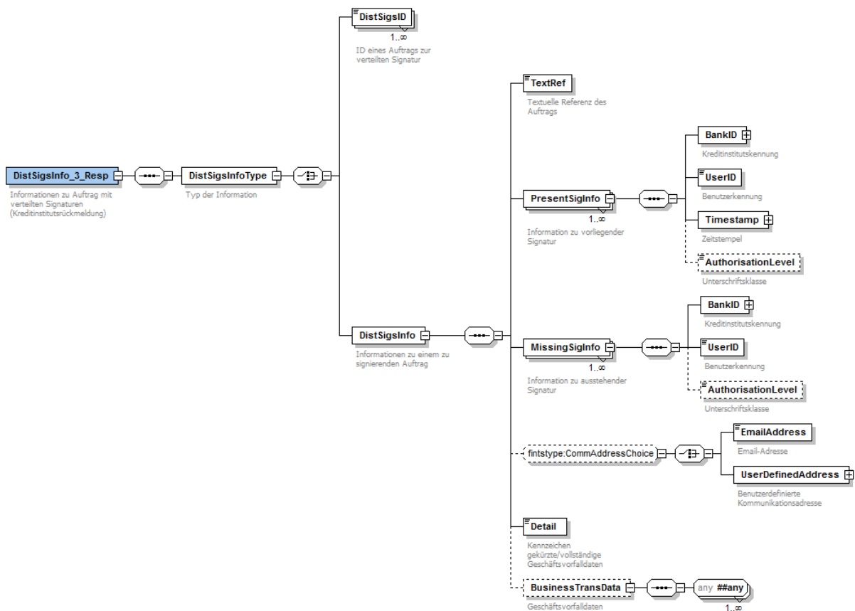
Abbildung 122: Kreditinstitutsrückmeldung Informationen zu Auftrag mit verteilten Signaturen
