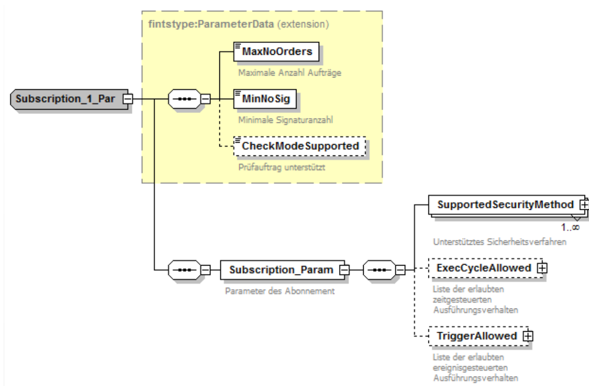
Abbildung 99: Bankparameterdaten Abonnement einreichen
