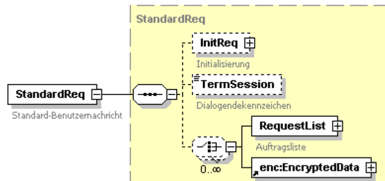
Abbildung 150: Auftragsverschlüsselung in der Standard-Benutzernachricht
