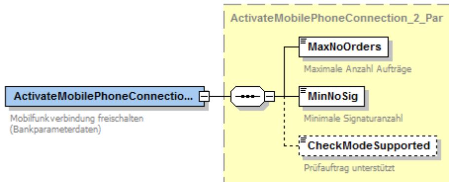
Abbildung 92: Bankparameterdaten Mobilfunkverbindung freischalten
