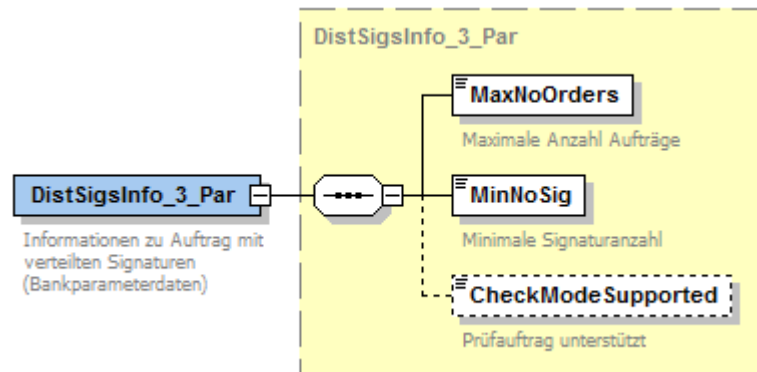
Abbildung 123: Bankparameterdaten Informationen zu Auftrag mit verteilten Signaturen
