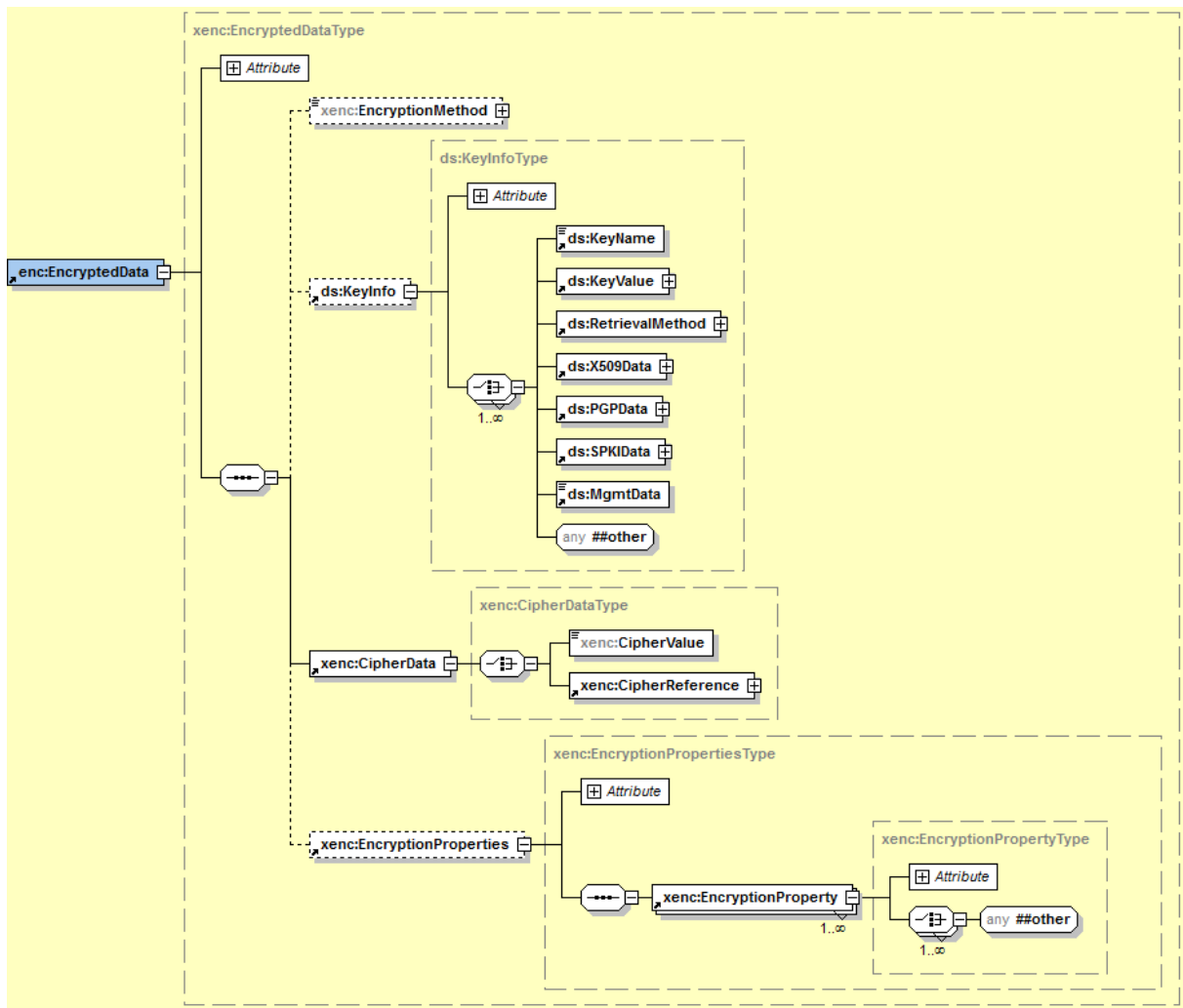
Abbildung 146: Verschlüsselung mit dem EncryptedData-Element
