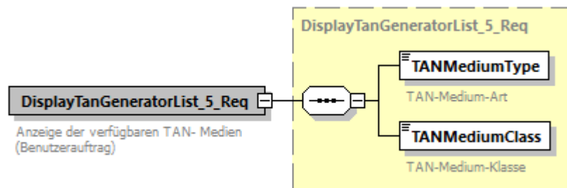
Abbildung 82: Benutzerauftrag Anzeige der verfügbaren TAN-Medien
