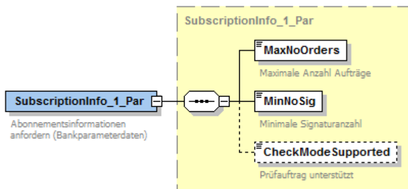
Abbildung 105: Bankparameterdaten Abonnementsinformationen anfordern
