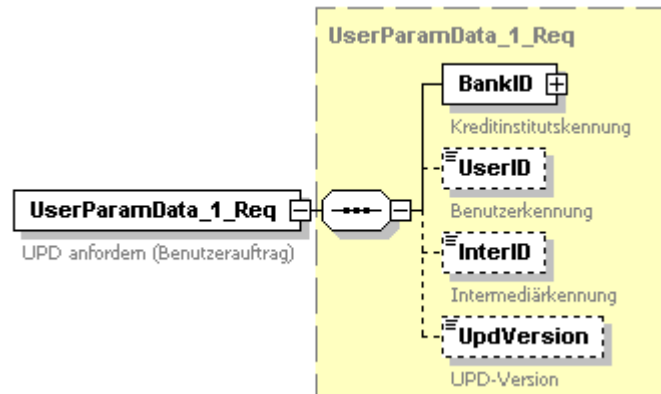
Abbildung 61: Benutzerauftrag UPD anfordern
