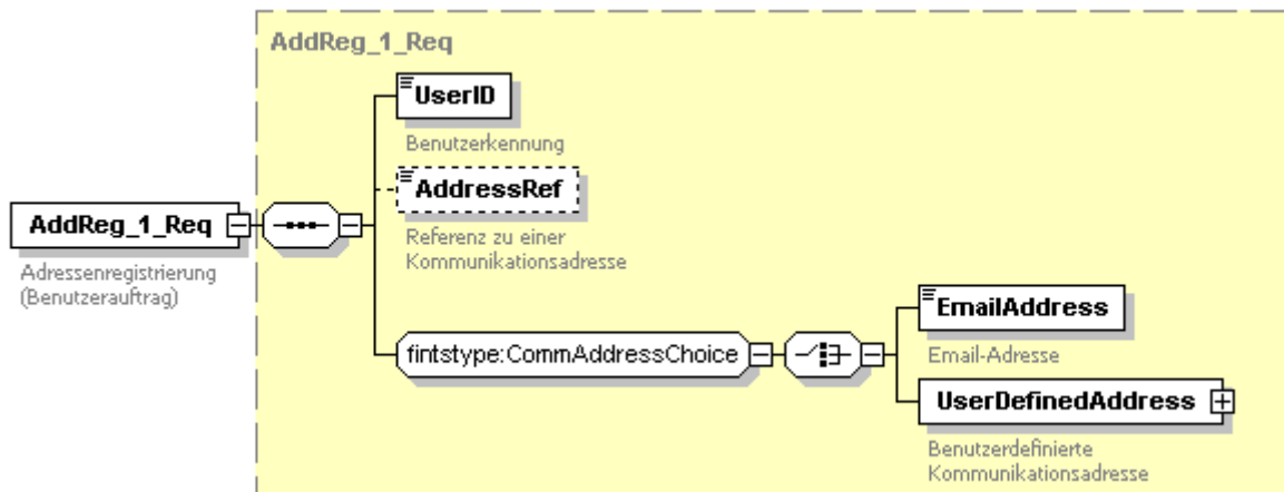
Abbildung 106: Benutzerauftrag Adresse registrieren
