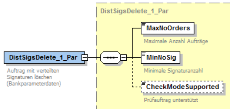
Abbildung 128: Bankparameterdaten Auftrag mit verteilten Signaturen löschen
