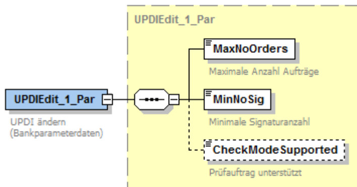
Abbildung 72: Bankparameterdaten UPDI ändern
