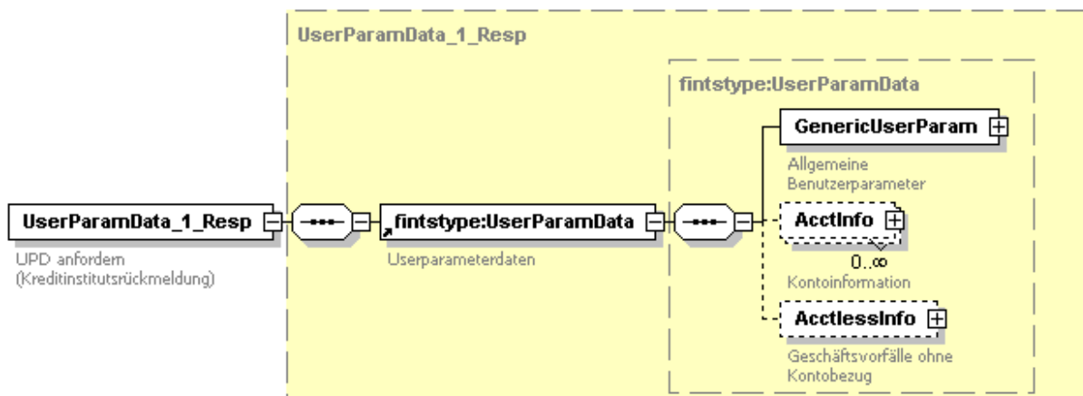
Abbildung 62: Kreditinstitutsrückmeldung UPD anfordern
