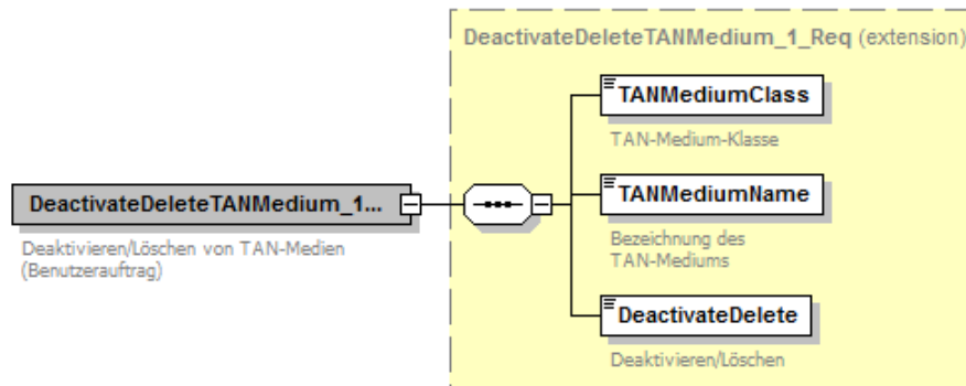
Abbildung 95: Benutzerauftrag Deaktivieren / Löschen von TAN-Medien
