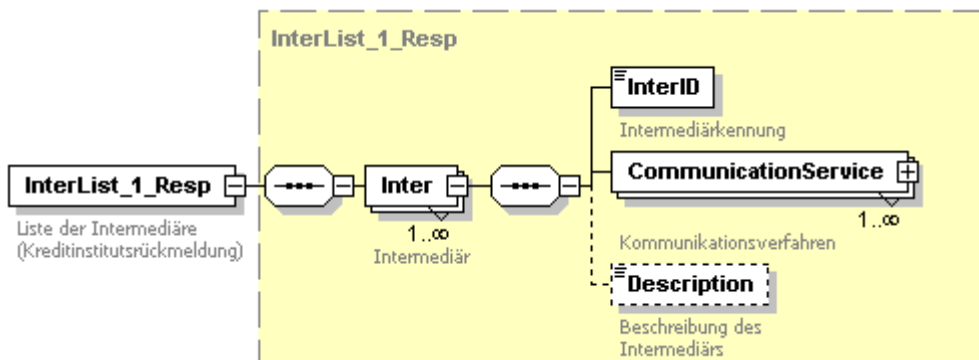
Abbildung 65: Kreditinstitutsrückmeldung Liste der Intermediäre
