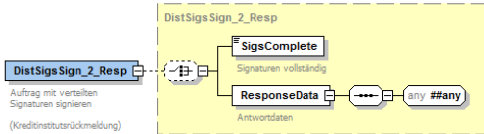
Abbildung 125: Kreditinstitutsrückmeldung Auftrag mit verteilten Signaturen signieren
