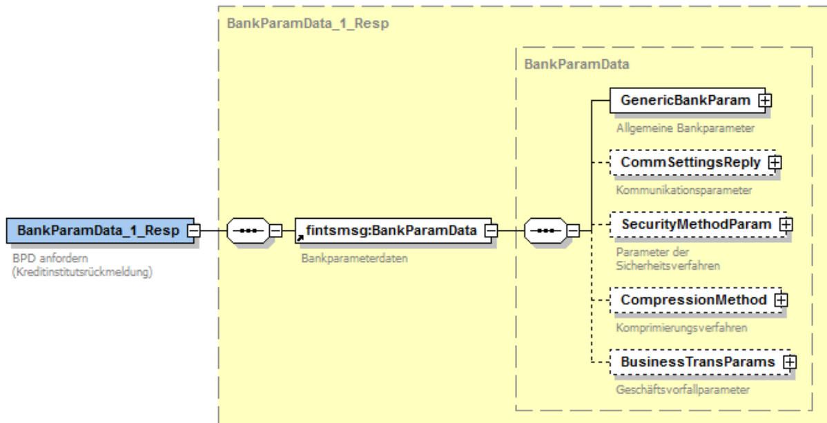
Abbildung 59: Kreditinstitutsrückmeldung BPD anfordern
