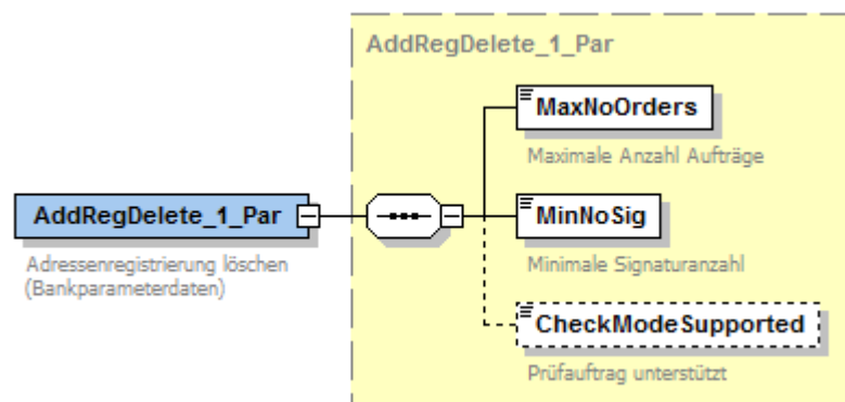
Abbildung 113: Bankparameterdaten Adressregistrierung löschen
