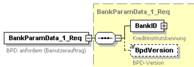
Abbildung 58: Benutzerauftrag BPD anfordern
