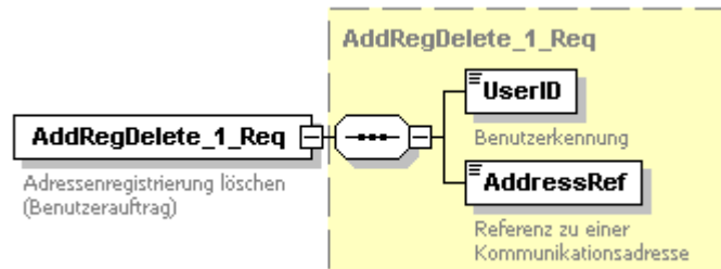
Abbildung 112: Benutzerauftrag Adressregistrierung löschen
