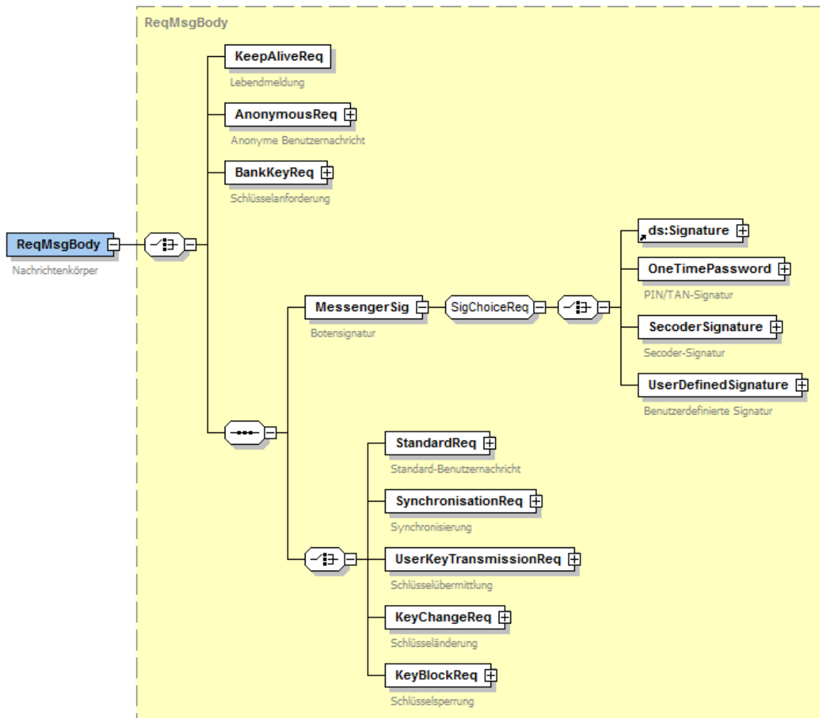
Abbildung 142: Botensignatur im Nachrichtenkörper einer Benutzernachricht
