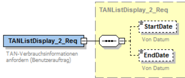
Abbildung 79: Benutzerauftrag TAN-Verbrauchsinformationen anzeigen
