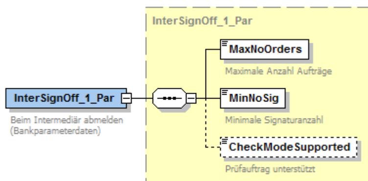
Abbildung 70: Bankparameterdaten Für einen Intermediär abmelden
