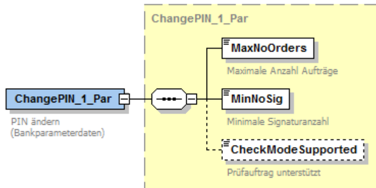
Abbildung 74: Bankparameterdaten PIN ändern
