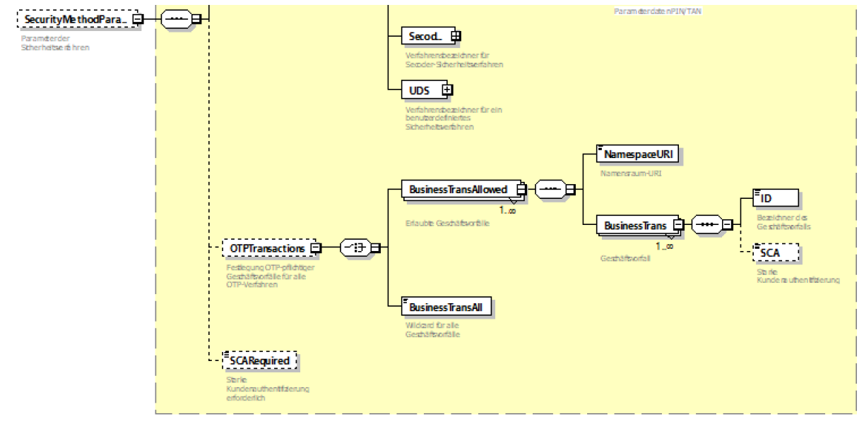
Abbildung 46: Festlegung OTP-pflichtiger Geschäftsvorfälle für alle OTP-Verfahren
