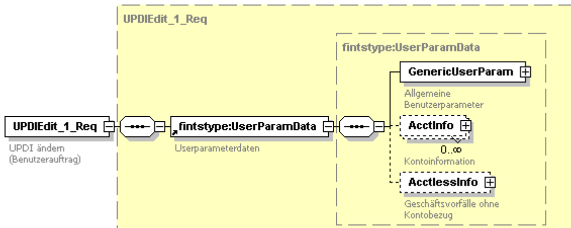
Abbildung 71: Benutzerauftrag UPDI ändern
