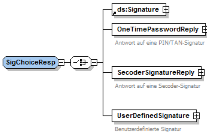
Abbildung 133: Signatur einer Kreditinstitutsnachricht
