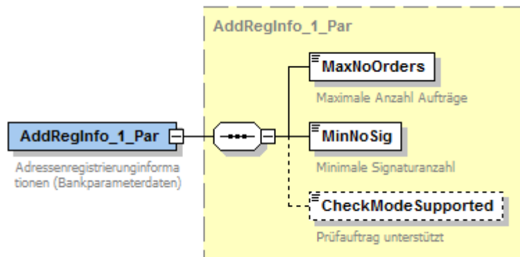
Abbildung 111: Bankparameterdaten Adressregistrierungsinformationen holen
