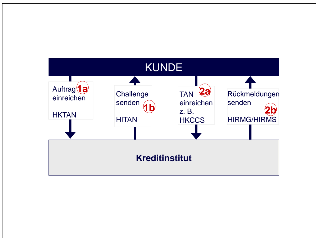
Abbildung 1: Abfolge der Operationen bei FinTS Prozessvariante 1
