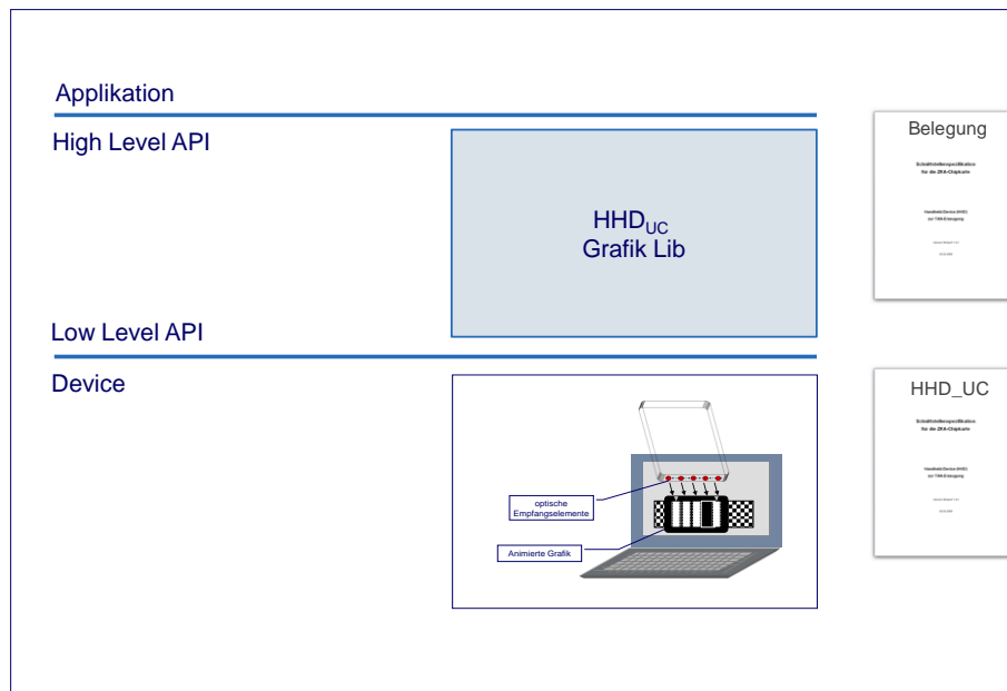
Abbildung 2: Definition der HHDUC-Anwendungsschnittstelle am Beispiel der animierten Grafik
